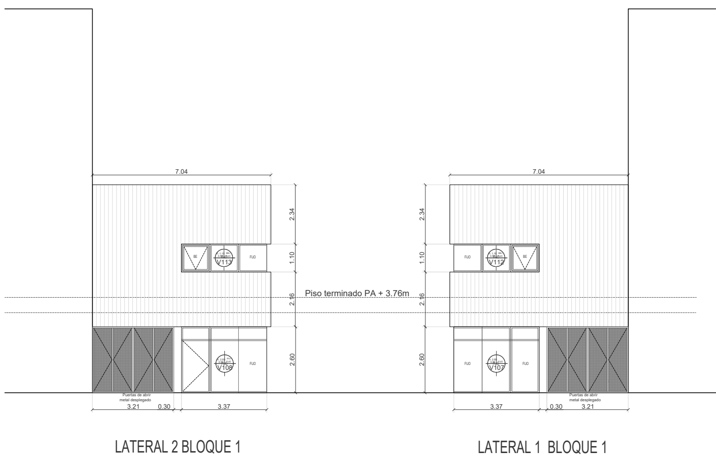
LATERAL 2 BLOQUE 1
