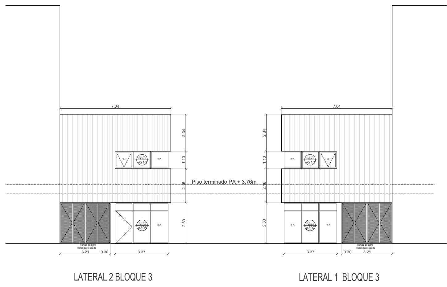
LATERAL 2 BLOQUE 3
