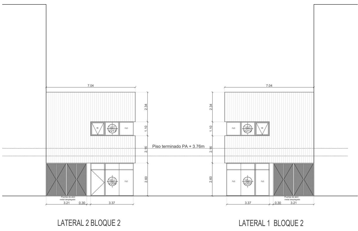
LATERAL 2 BLOQUE 2
